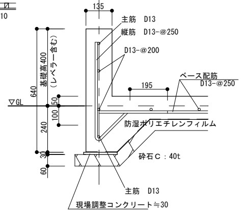
基礎断面図 S=1:20
