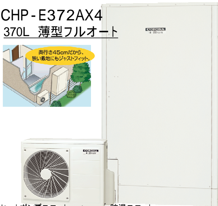
ヒートポンプユニット CHP-4516 幅900×奥行300×高さ650mm 貯湯ユニット CTU-E372AX4 幅1,090×奥行450×高さ1,890mm
