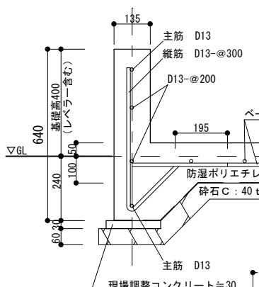
基礎断面図 S=1:20
