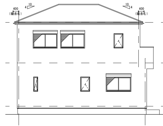
西側立面図 S=1:150
