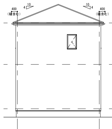
北側立面図 S=1:150
